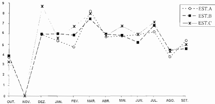
Figura 3 - Taxa de Oxigênio dissolvido (ml/l) na água intersticial durante o período de amostragens.
